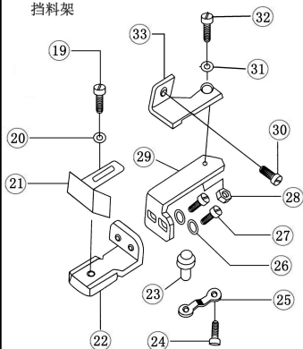
796 专用 挡料架
